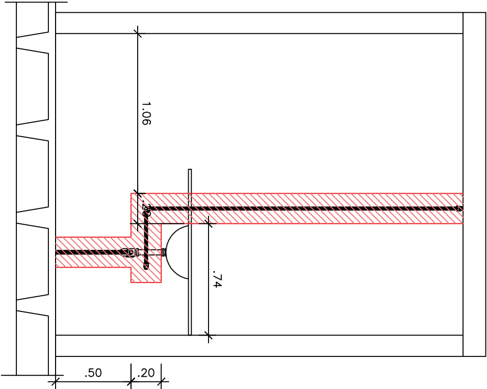
Vista J ESCALA 1/25
