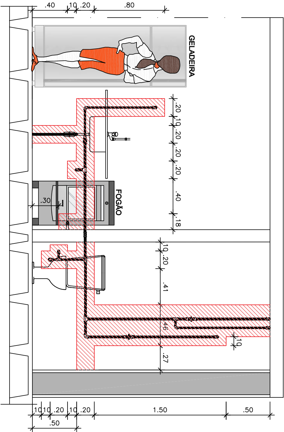
Vista I ESCALA 1/25
